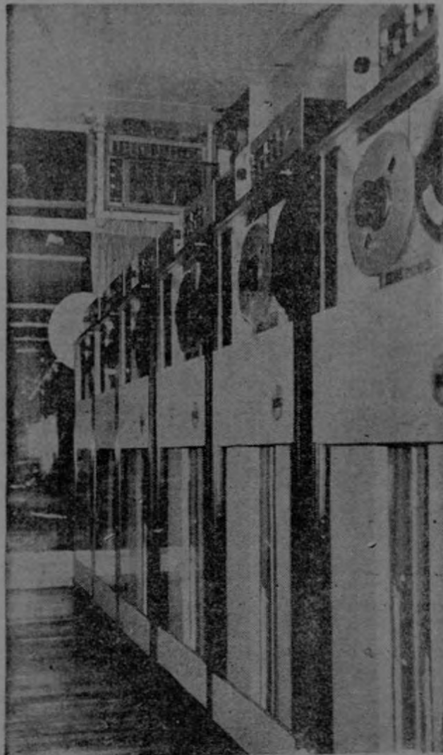
Unidades de cinta magnética MAI para grabación y lectura de datos a la velocidad de 60.000 caracteres por segundo.
